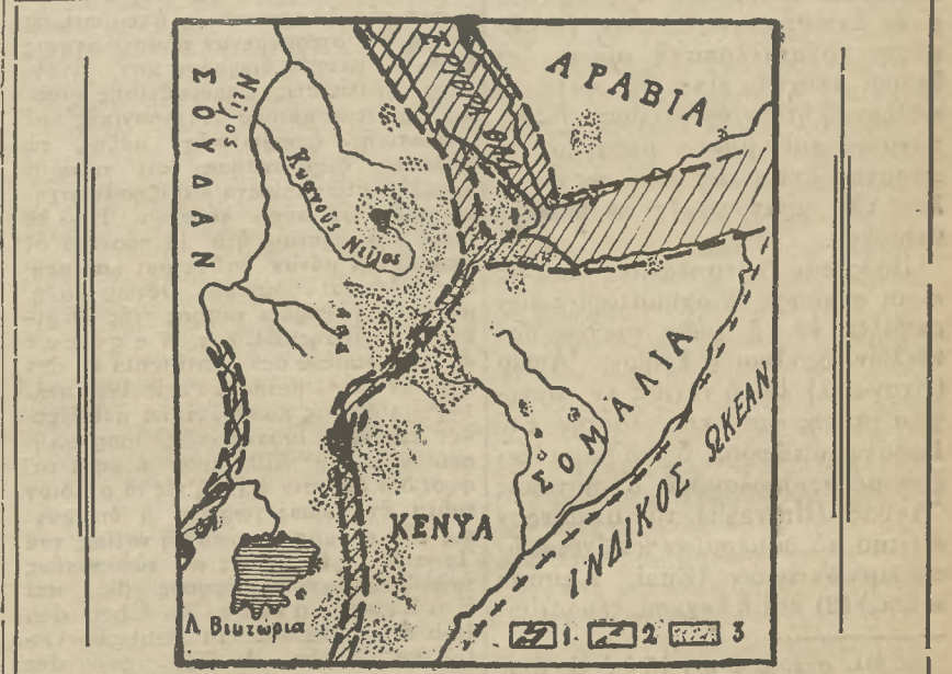
Μεγάλοι τεκτονικοί γραμμάι έν 'Αιθιοπία και ταίς γειτονικάίς χώραις. 1=Μεγάλοι τάφροι, 2=Άλλαι ηη-ξίγενείς γραμμάι, 3=Ήφαιστειογενή πετρώματα.
